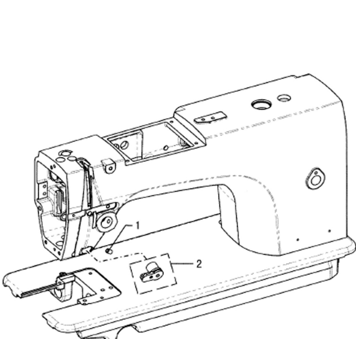
9. 夹线装置/WIRE CLAMPING DEVICE
