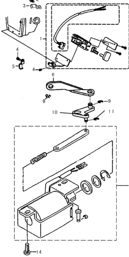
8. 自动倒缝装置/AUTOMATIC REVERSE MECHANISM
