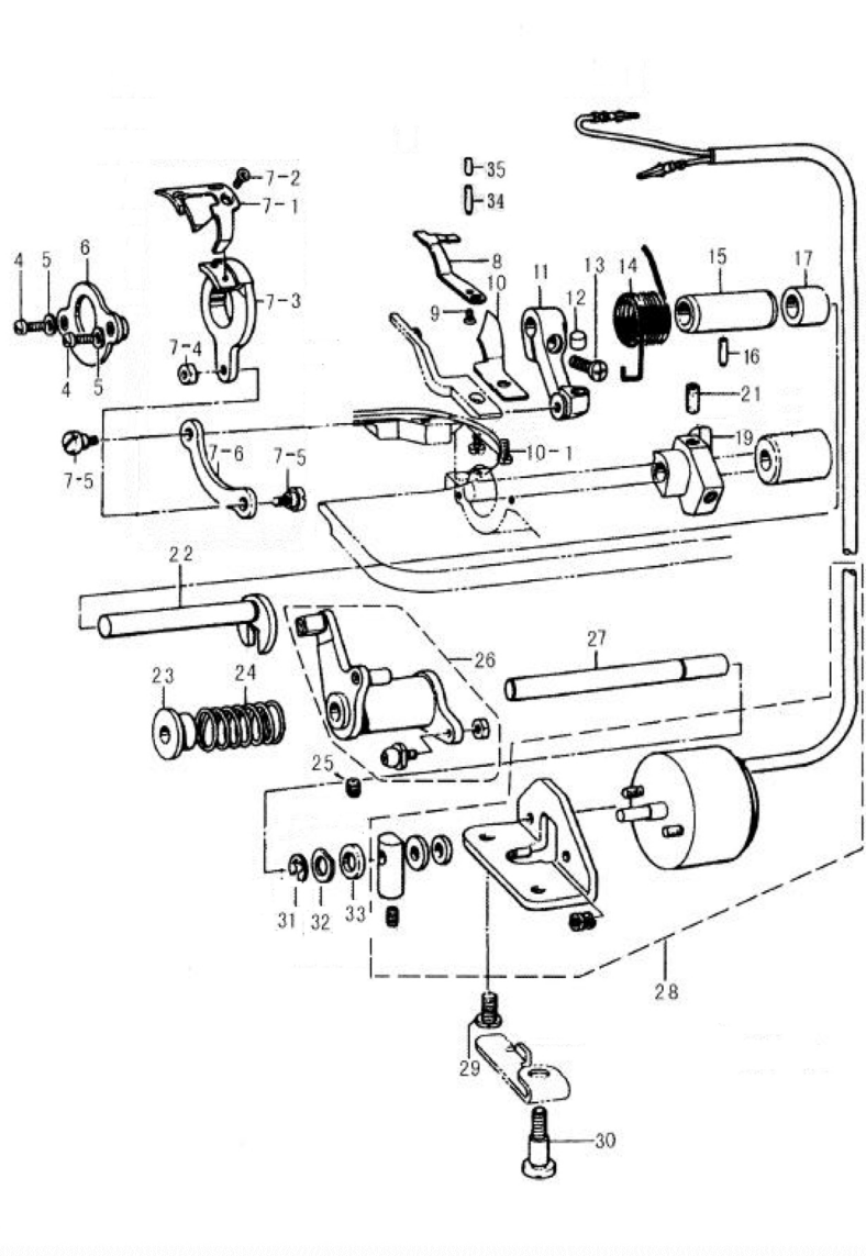
7. 自动切线装置/THREAD TRIMMER MECHANISM
